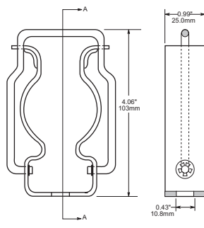
270303 DIN Fuseclip
